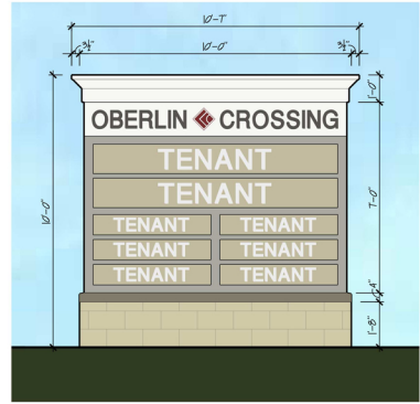
MONUMENT SIGN SCALE: 3/8" = 1'-0"
